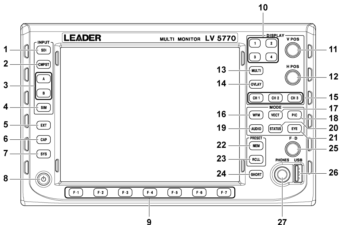
図 3-1 前面パネル
