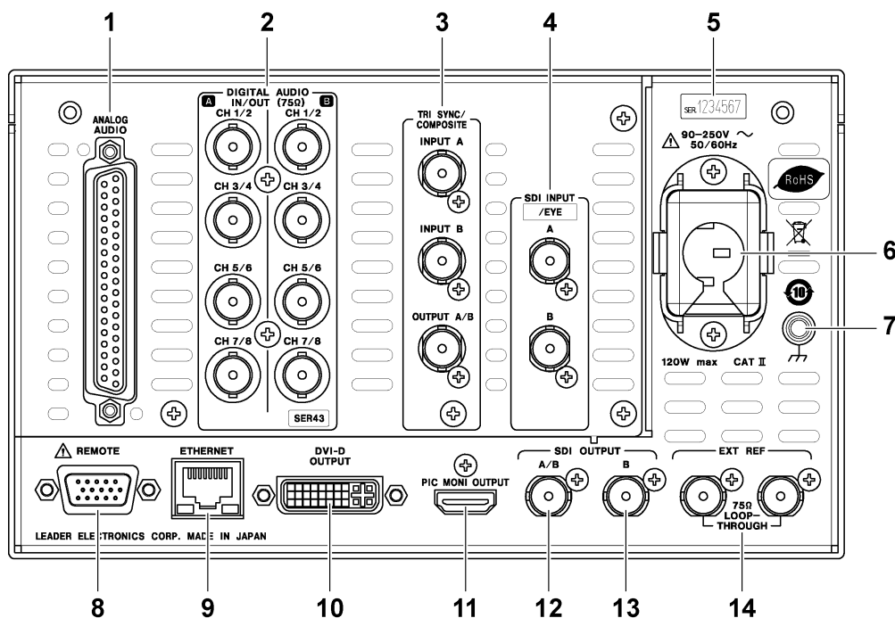
図 3-2 背面パネル
