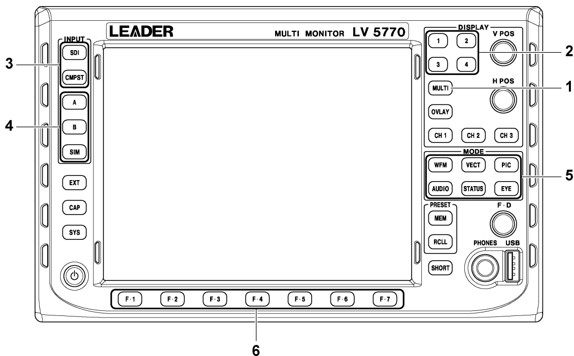
図 5-1 操作手順
