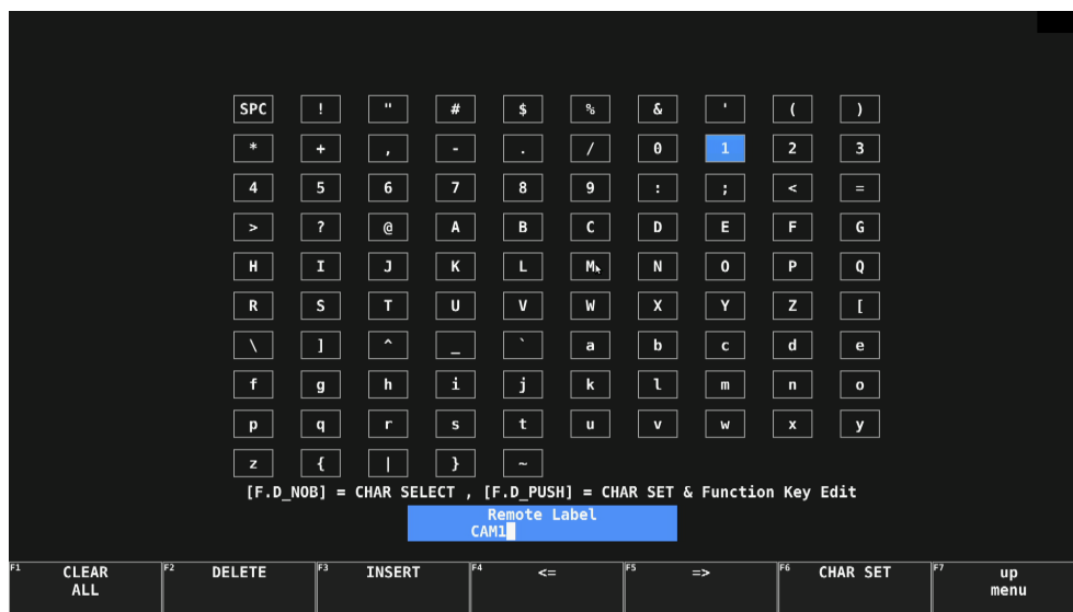
Figure 6-18 ラベル入力画面
