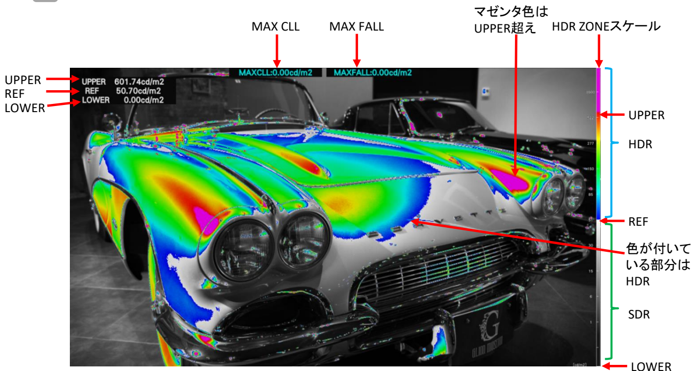
HDR ZONE表示
