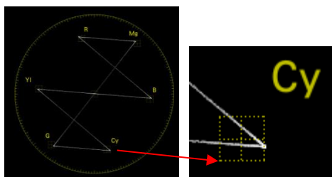
VECTOR SCALE BT.709設定 (ターゲットから外れています。)
